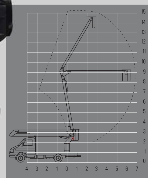
Diagrama de Alcances Hidralift 240/15
